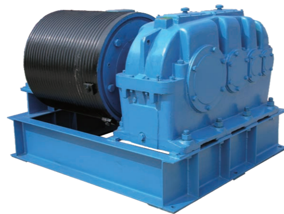
JK6吨电动快速卷扬机，用于山西福盛钢铁 公司石灰窑上料用。
