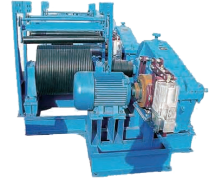
JK3吨石灰窑上料卷扬机 用于新疆天业集团
