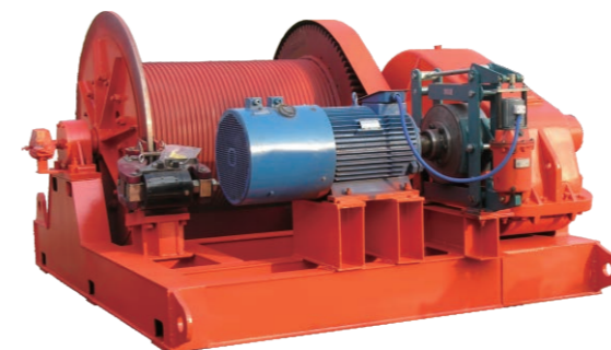
中铁二十二局450+450吨提梁机主起升用 JM13.5吨卷扬机 容绳量：380m 额定速度：5m/min
