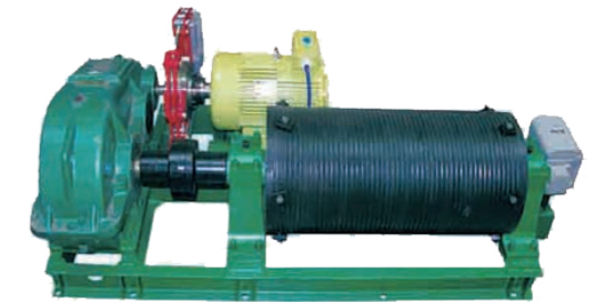
JK5吨电动快速料车卷扬机 用于邯郸钢铁公司石灰窑上料
