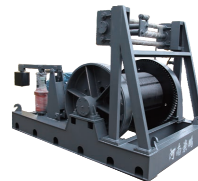
JK9吨快速卷扬机 绳速：30m/min 容绳量：650m
