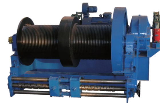
河南矿山75T-75m起重小车主起升用 JM2×10吨卷扬机 容绳量：2×350m 额定速度：10m/min
