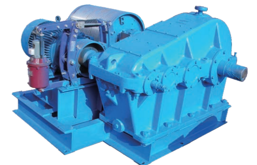
JK5吨卷扬机 用于洛阳矿业集团氧化钙上料
