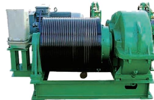
JK5吨电动快速料车卷扬机 用于霸州钢厂石灰窑上料
