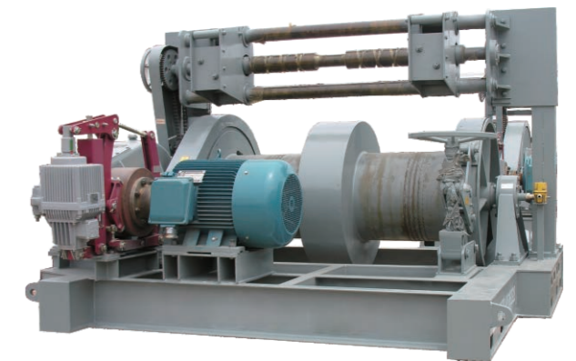
中海一号350t起重船用 2JK2011吨主提升绞车
