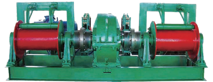
为洛阳热电厂烟囱检修工程配套2JK5卷扬机， ( F=50\text{KN} , V=20\text{m/min} , d=21.5\text{mm} , L=2 \times 220\text{m} ) 其结构特点：双绳起吊，安全：配压绳器，钢丝绳排列整齐。
