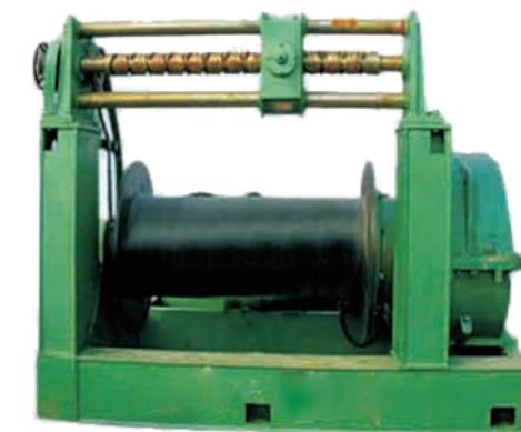
JK8吨电动快速卷扬机 用于MG80吨吊钩门式起重机主起升机构 (中国三峡总公司溪洛渡工程)
