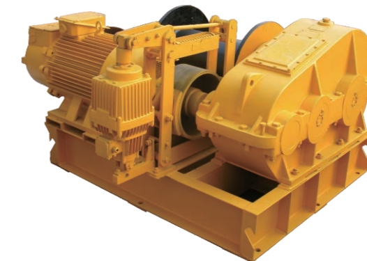
ZKL800-26螺旋钻机用 JK5吨卷扬机
