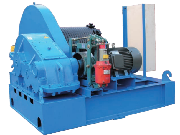
凌源钢厂380m高炉清炉渣用JM20T卷扬机 容绳量60m 额定速度6m/min
