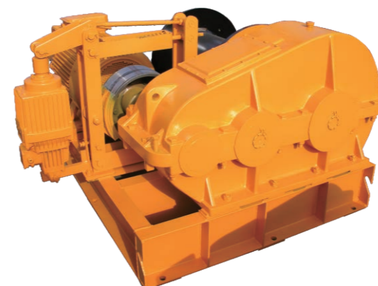
ZKL800-30螺旋钻机用 JK8吨卷扬机
