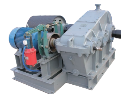
JK5吨快速卷扬机 绳速：49.2m/min 行程：40m 洛阳矿业集团纳米公司石灰窑上料用
