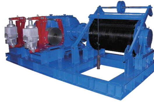
JK5.6吨石灰窑上料卷扬机 用于北京埃肯公司
