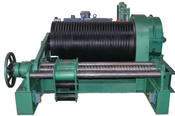
JM10吨变频调速卷扬机（带排绳器） 钢卷轧机生产线拉钢带用
