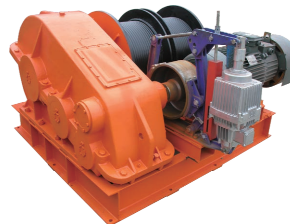
JK10吨电动快速卷扬机 用于MG40吨吊钩门式起重机主起升机构 (中铁十七局第三工程有限公司)
