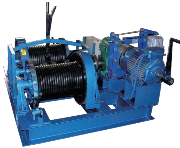
2JMW5吨卷扬机 焦化厂检修炉门专用
